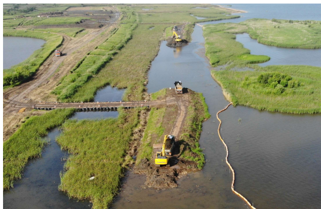
令和2年7月矢臼場河道掘削（石狩市）
